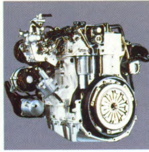
2068 cm 3 turbo dieselmotor
