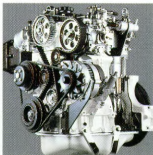
2068 cm 3 dieselmotor
