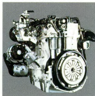
2068 cm 3 turbo dieselmotor
