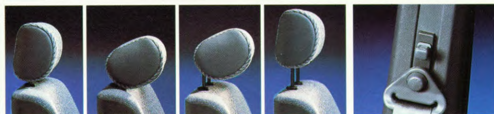
Verstelbare hoofdsteunen en in hoogte verstelbare bevestiging van de veiligheidsgordels.
