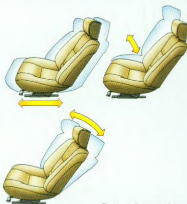
Bestuurdersstoel met verstelbare rugleuning en dicht naast elkaar geplaatste stelrails, in hoogte verstelbaar.
