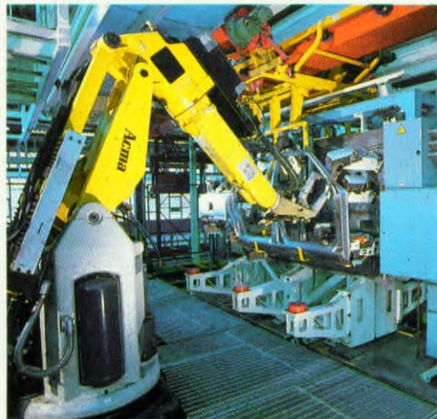
2. Robot lasstraat
