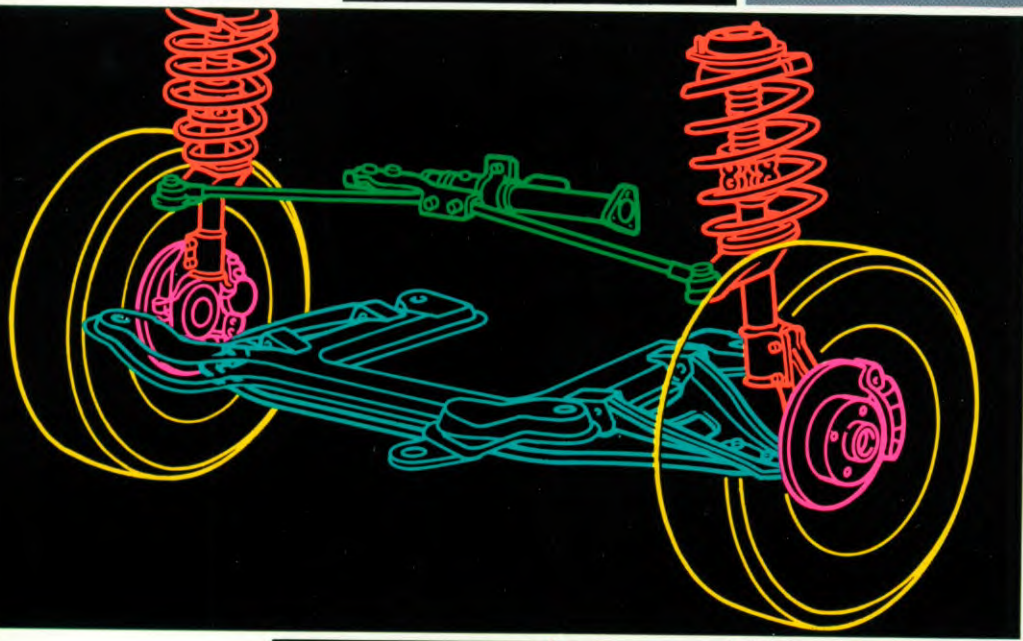
Mac Pherson voortrein met negatieve stuurstraal
