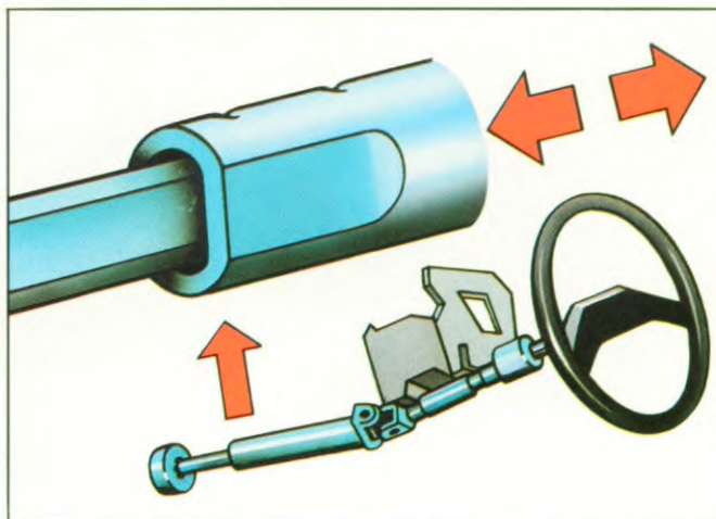
Telescopische stuurkolom met kruiskoppeling verhindert binnendringen van stuur.
