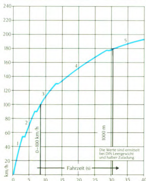
Beschleunigungsdiagramm Schaltgetriebe
