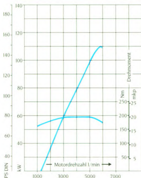
Vollastkurven
