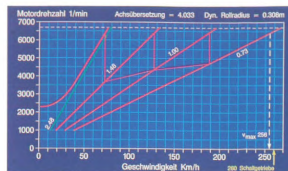
Die Getriebeabstufung optimiert in Verbindung mit dem intelligenten Schaltprogramm der Porsche Tiptronic den Beschleunigungsverlauf des 911 Carrera 2
