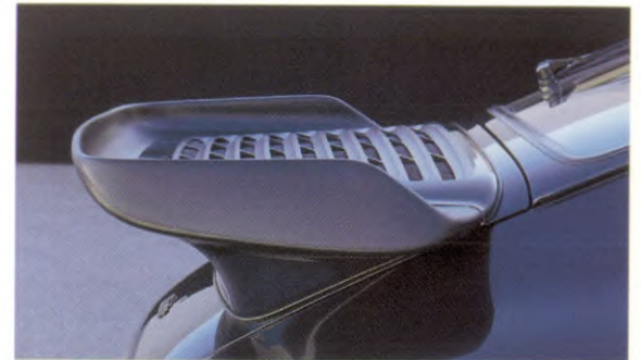
Charakteristische, breite Turbo Heckpartie. In den feststehenden Spoiler ist der Ladeluftkühler integriert
