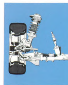
Die Vorderräder werden an Dreieckslenkern und Federbeinen geführt
