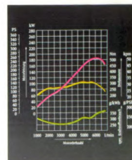
Gleichmäßiger Leistungsanstieg bis zum Erreichen der Nenndrehzahl
