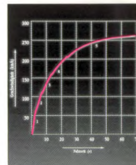
Die Beschleunigung des 911 Carrera 4 weist ihn als Spitzensportler aus
