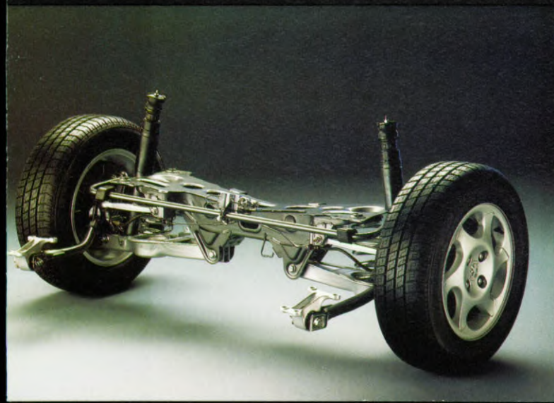
► De multi-link achtertrein met fractioneel meesturende achterwielen.
