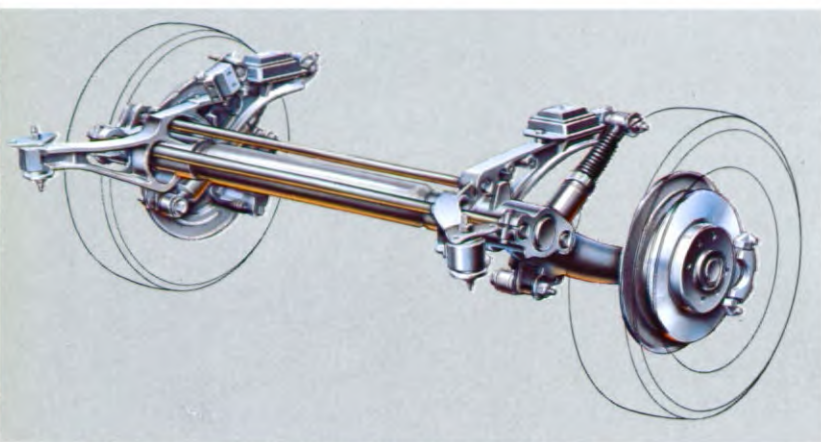
Achtertrein met horizontaal geplaatste schokdempers.
