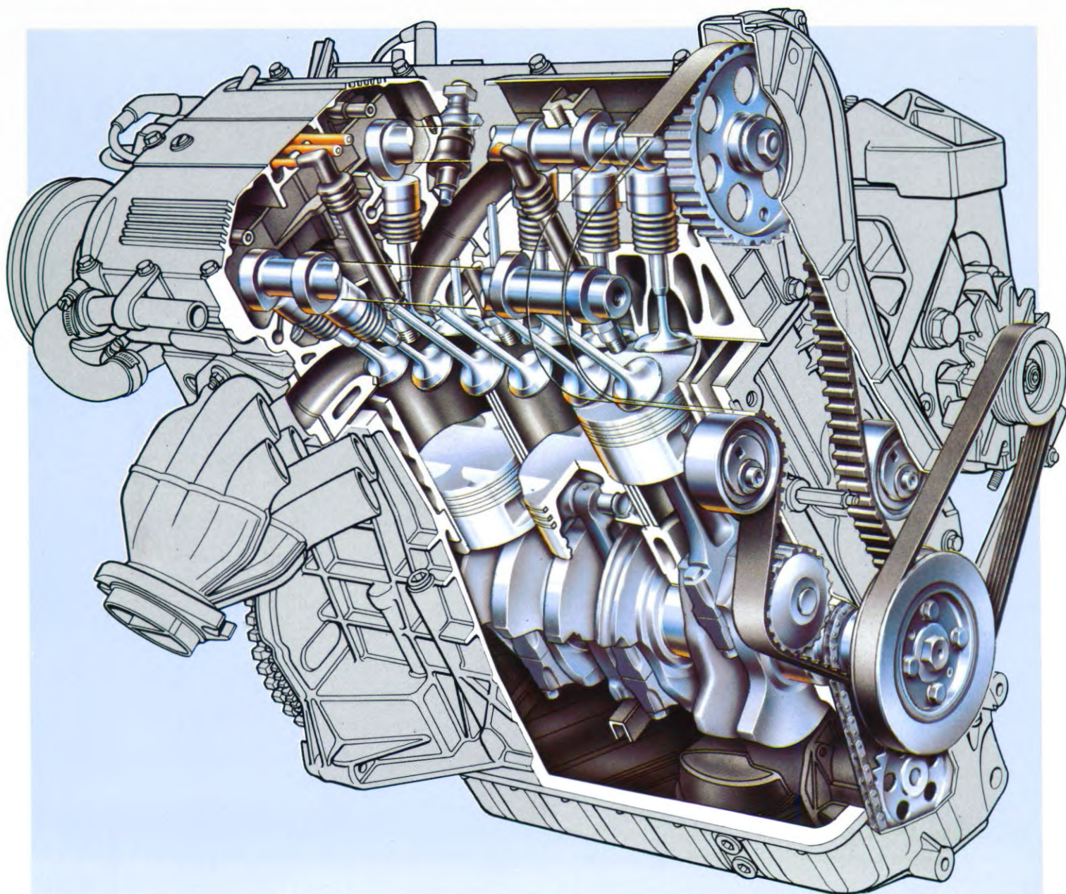
1905 cm 3 16-kleppen benzine-injectiemotor.
