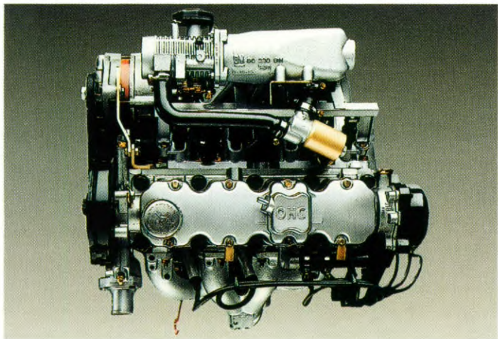
De 2.0i-motor met 85 kW (115 DIN-pk) en geregelde 3-weg-katalysator.
