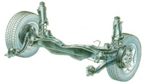
De nieuwe "multi link"-achterwielophanging van de Vectra staat borg voor
