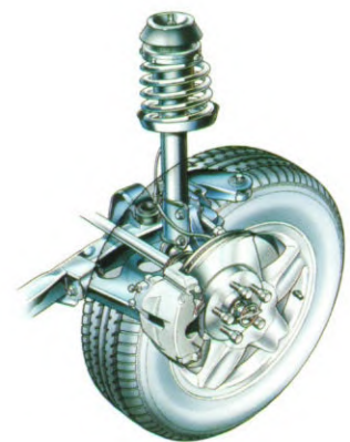
De "Dynamic Safety"-voorwielophanging zorgt voor optimale besturing en een betere remstabiliteit.
