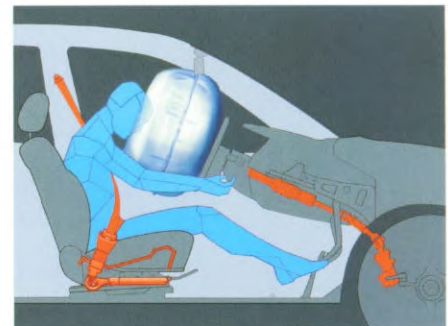
De telescopische stuurkolom vermindert het gevaar dat deze bij een frontale aanrijding in de cabine dringt. De
