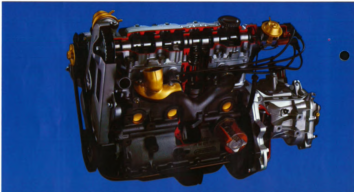
1.3 l OHC-motor.
