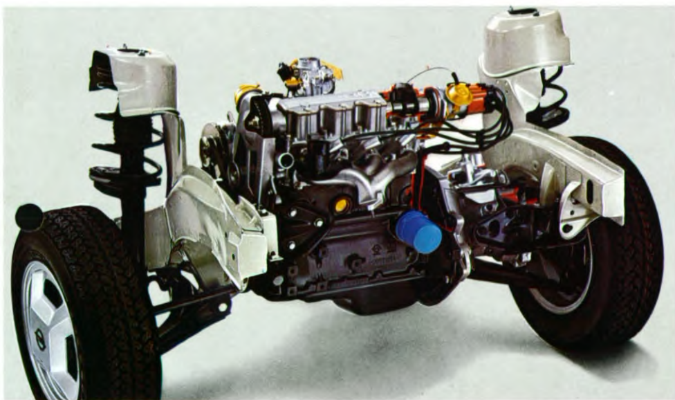
Aandrijvingseenheid.
