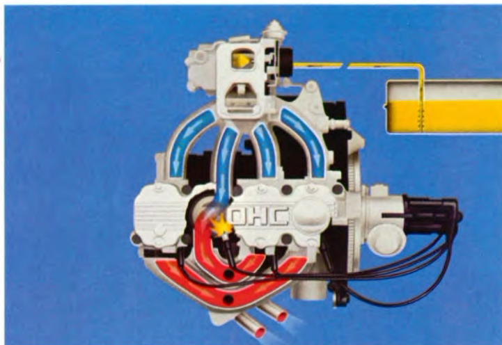
Brandstofbesparend dwarsstroomprincipe.
