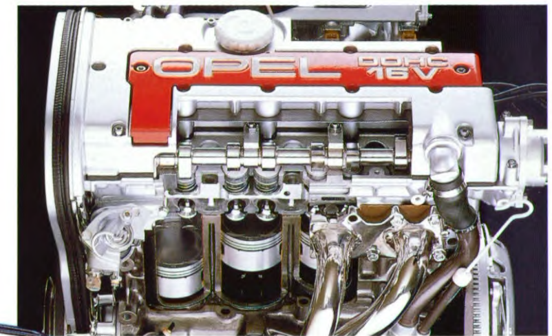
2.0i-16-kleppenmotor.
