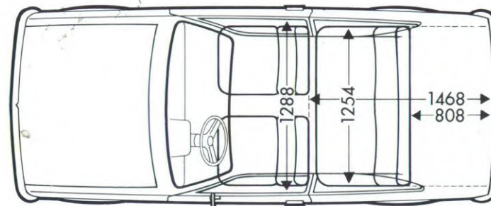
Schouderhoogte vóór 1288 mm, laadruimbreedte vóór 1254 mm, laadvloerlengte tot achterzijde zitting 808 mm, laadvloerlengte tot achterzijde voorstoel 1468 mm.
