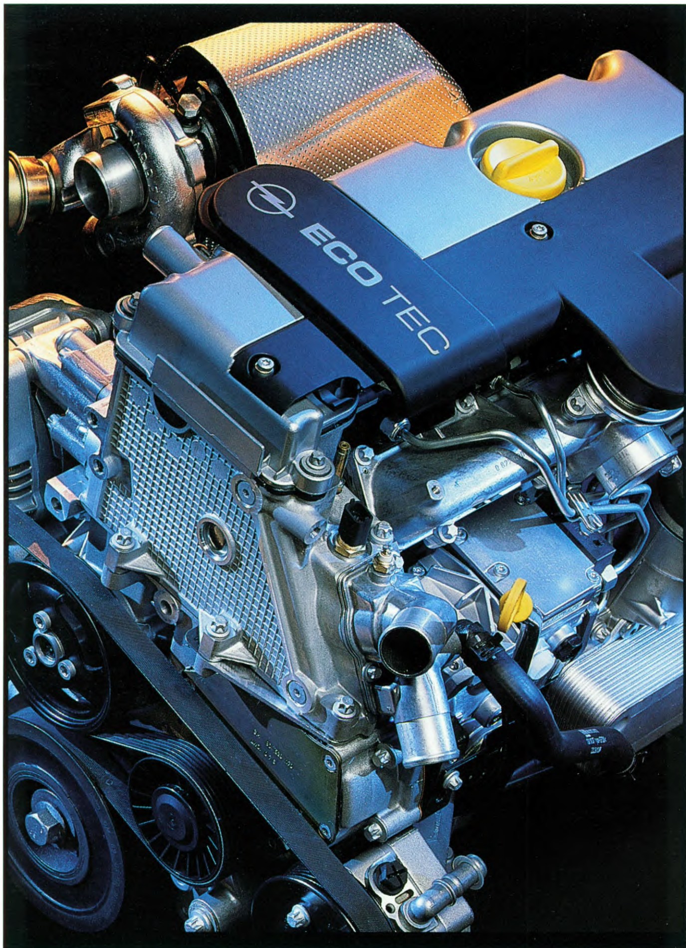
4-kleppentechniek en directe inspuiting gecombineerd in een Turbodiesel: de nieuwe 2.0-DTI-16V (74 kW/100 DIN-pk).
