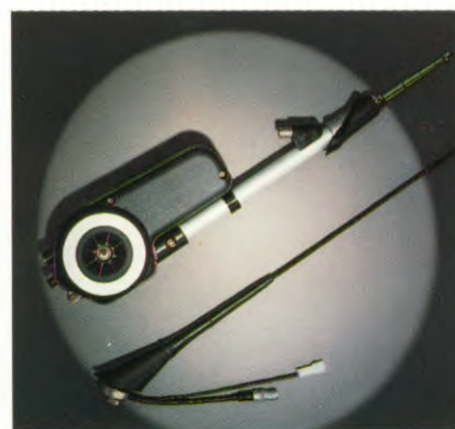
Motorantenne , (niet afgebeeld) voor montage achterop.
