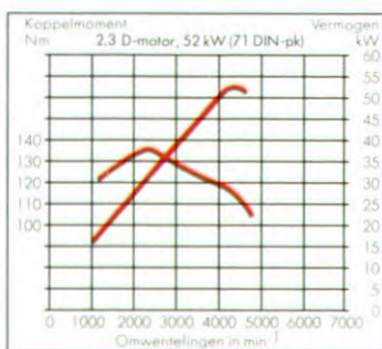
2.3 Diesel-OHC-motor. 52 kW (71 DIN-pk) bij 4400 min -1 . Bovenliggende nokkenas.
