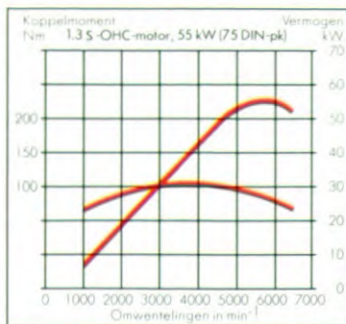
1.3 S-OHC-motor. 55 kW (75 DIN-pk) bij 5800 min -1 . Bovenliggende nokkenas, hydraulische klepspelingsregeling, elektronische ontsteking.
