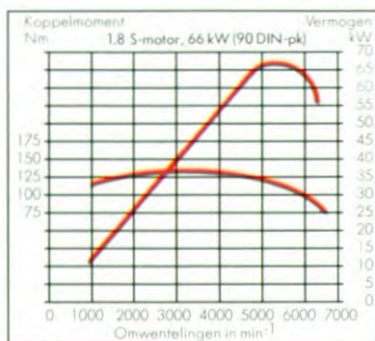
1.8 S-OHC-motor. 66 kW (90 DIN-pk) bij 5400 min -1 . Bovenliggende nokkenas, hydraulische klepspelingsregeling, elektronische ontsteking.
