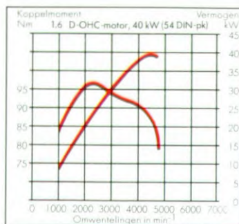
1.6 Diesel-OHC-motor. 40 kW (54 DIN-pk) bij 4600 min -1 . Lichtmetalen cilinderkop, bovenliggende nokkenas, hydraulische klepspelingsregeling.
