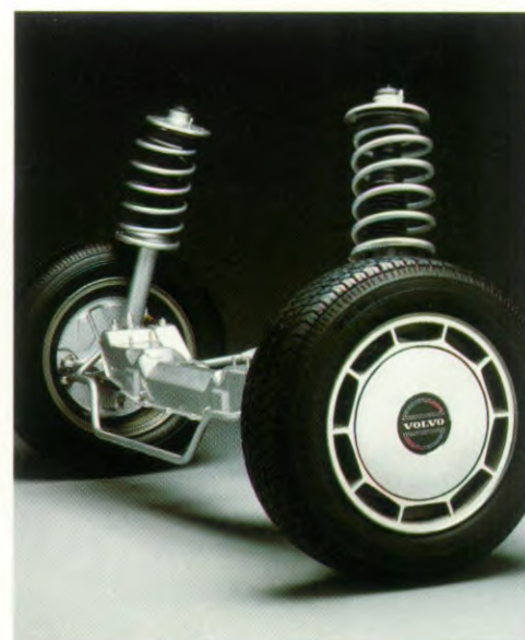
Tandheugelstuurinrichting. McPherson veerpoten.
