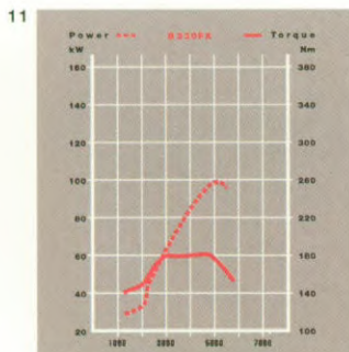
TURBO PLUS
