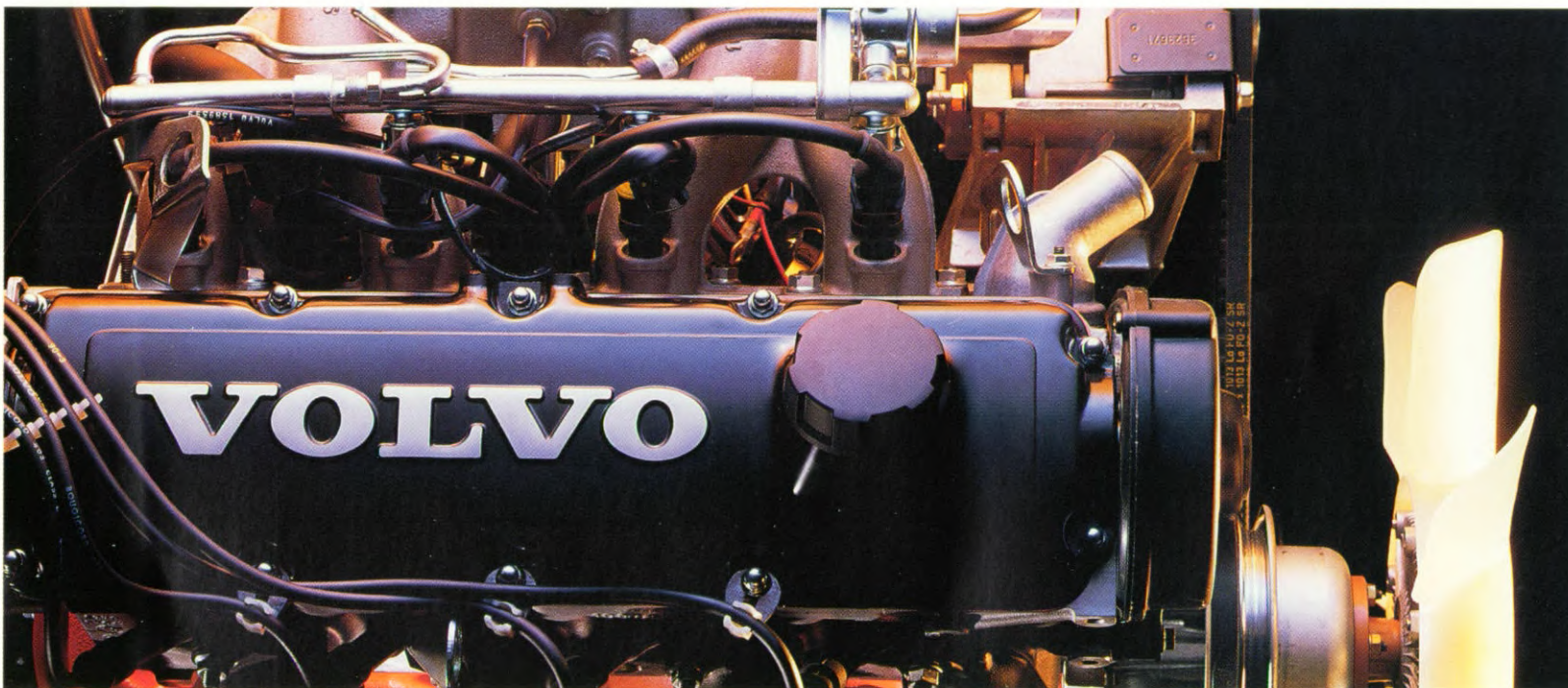
Volvo 2.3 liter injectiemotor met Lambdasonde.
