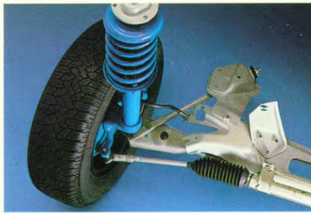
Onafhankelijke McPherson voorpoten.
