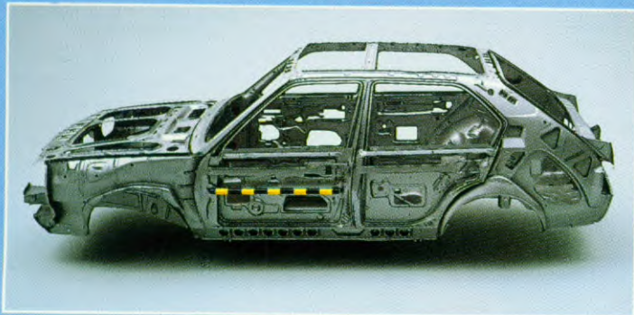
Een stalen veiligheidskooi en ingebouwde stalen buizen in de voorportieren voor extra bescherming.
