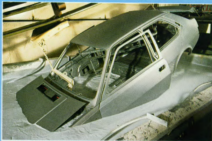
Onderdompeling in een cataforese-bad om de auto te voorzien van een optimale anti-roestbescherming.
