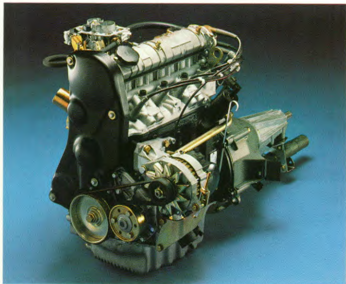
De Volvo 1.7-liter motor. Een krachtige nieuwkomer.
