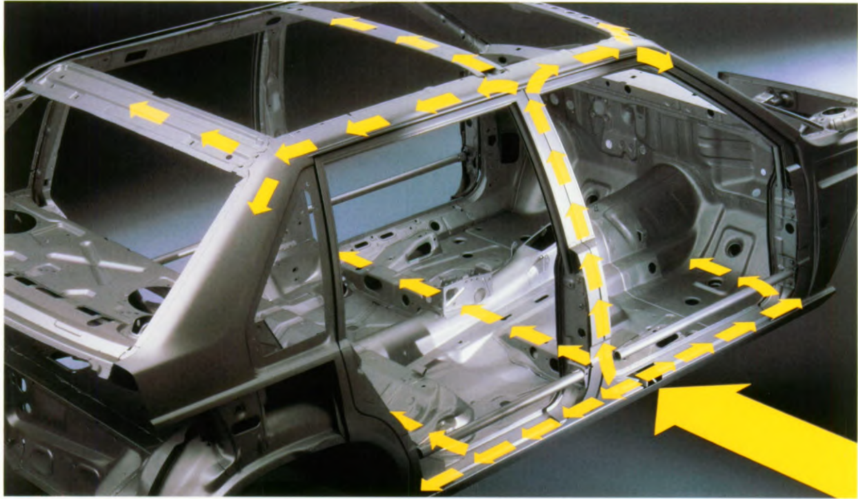
Volgens het SIPS-principe worden bij een zijdelingse botsing de krachten geabsorbeerd en verdeeld over de verschillende delen van de auto, waardoor een botsing beter kan worden opgevangen.
