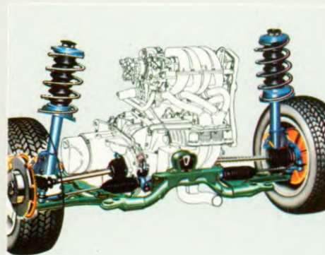
Voorwielopanging.
