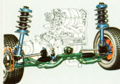
Voorwielloophanging.
