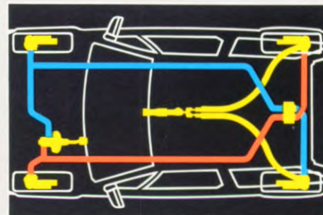
Diagonaal gescheiden remsysteem.
