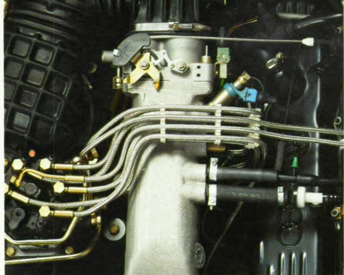
Het injectiesysteem van de vijfcilinder motor
