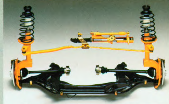
Vooras met McPherson voorpoten.
