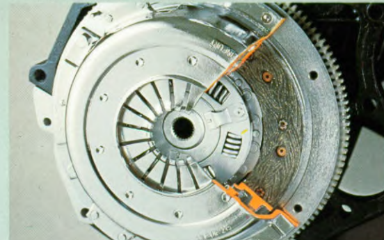
De hydr. bediende enkelvoudige droge plaatkoppeling van de 5 cilinder motoren.
