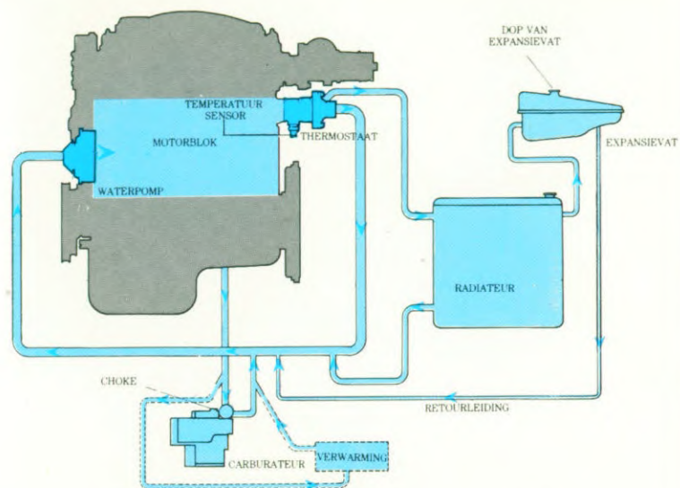
KOELSYSTEEM VAN DE SEAT MOTOR SYSTEM PORSCHE
